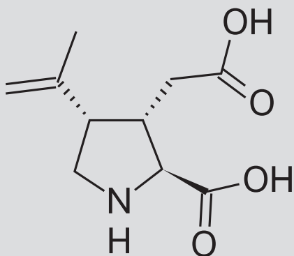
Рис. 5. Химическая структура каиновой кислоты
