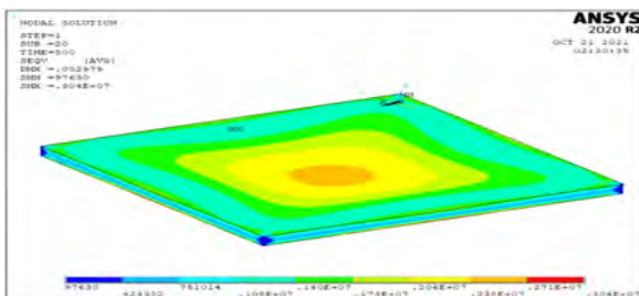
Рис. 2. Распределение напряжений по поверхности пластины, Па
