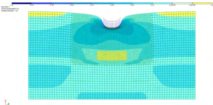
Рисунок 5 – Изополя распределения распорных напряжений
