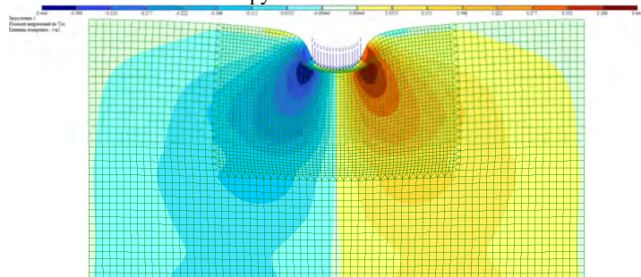
Рисунок 3 – Теоретическое описание распределения нормальных напряжений грунтовым массиве
