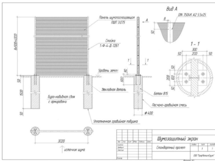
Рис. 1 - Шумопоглощающий экран
