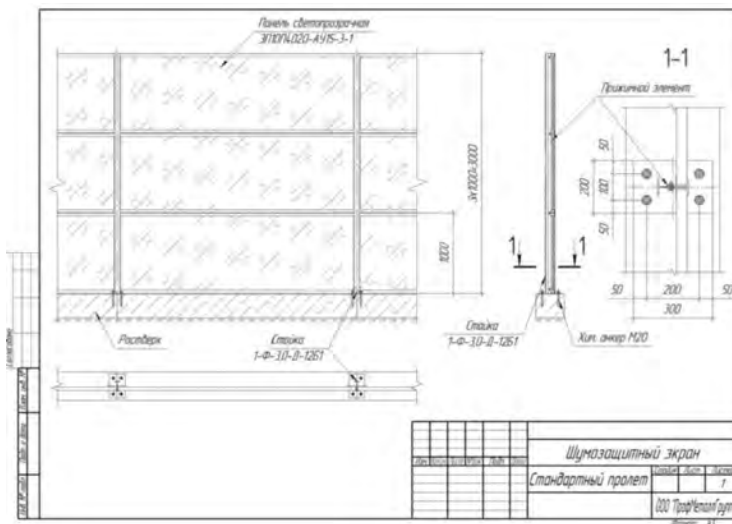
Рис. 1. Шумоотражающий экран
