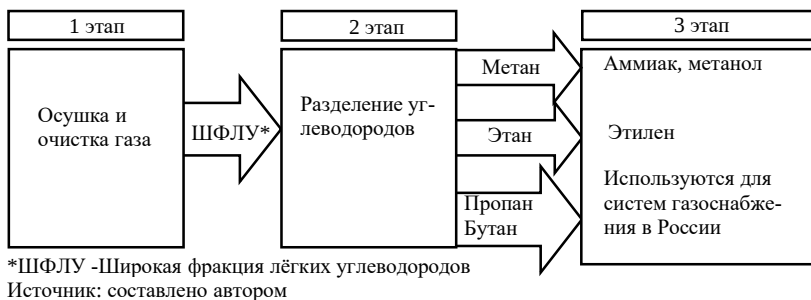
Рисунок 1. Основные этапы процесса газохимии
